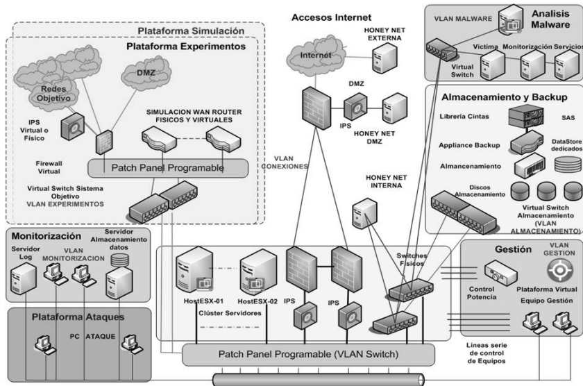
Figura 1. Diagrama lógico Infraestructura Experimentación
