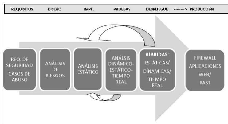
Figura 3. Modelo ciclo vida del software
