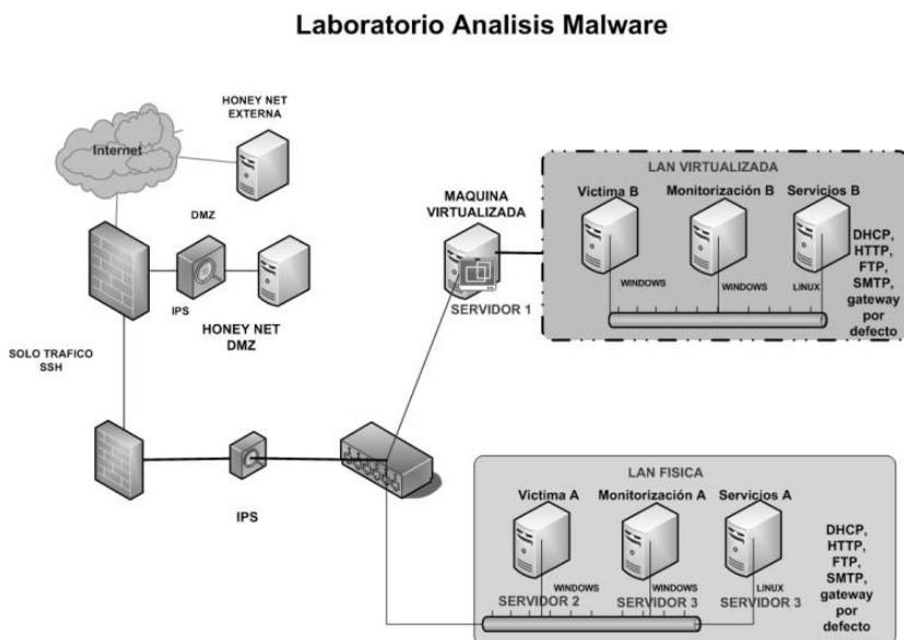
Figura 5. Diagrama laboratorio análisis malware
