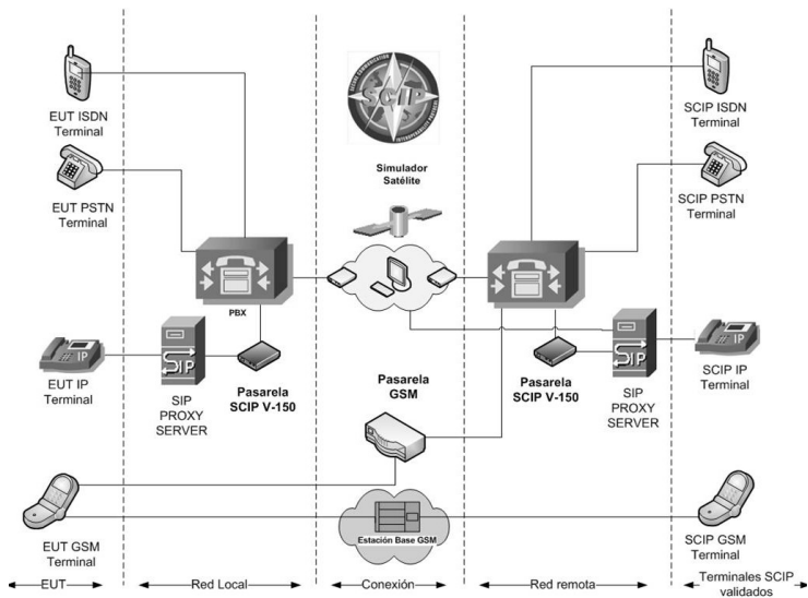
Figura 4 Banco de pruebas interoperabilidad SCIP
