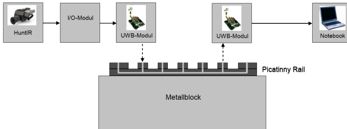
Figura 1 Sistema UWB para la comunicación de señales arma-soldado
